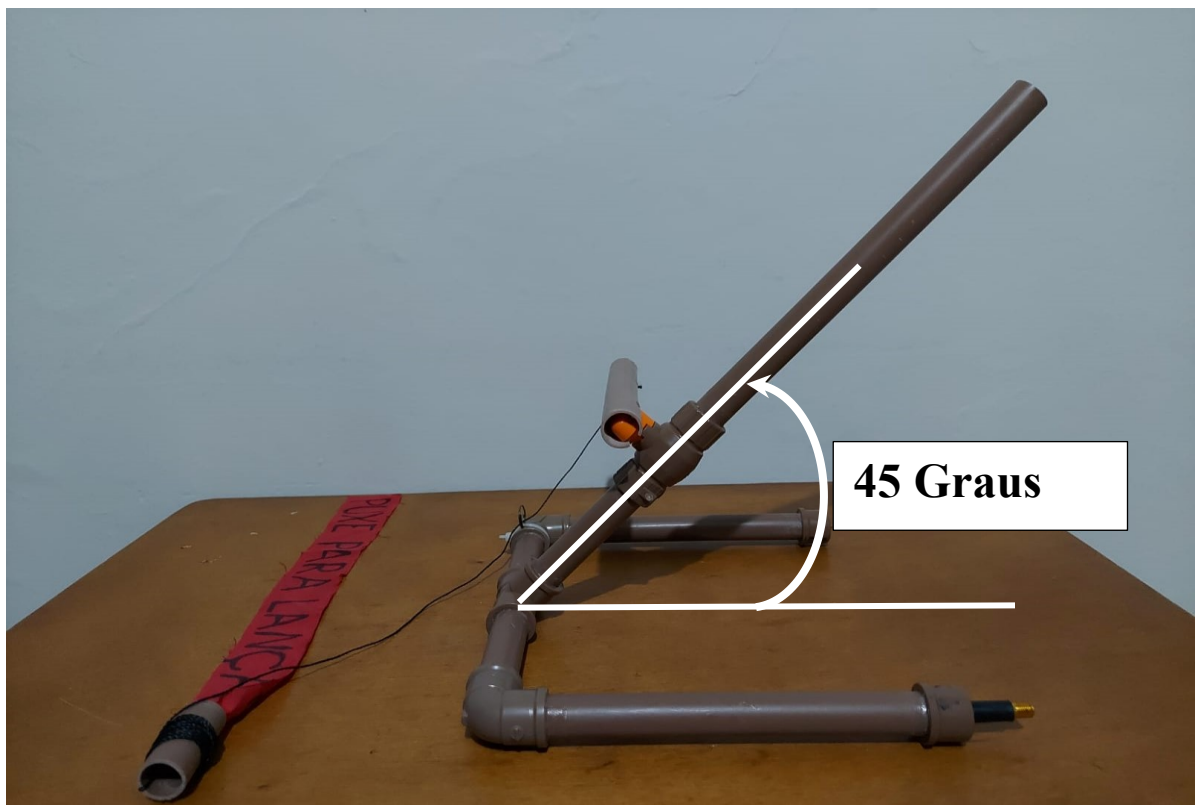
Vista lateral da base de lançamento do foguete no nível 1, mostrando a inclinação de 45 graus do tubo de lançamento.
