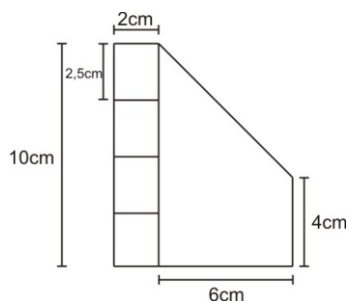
Figura 2. Dimensões e formato da aleta
